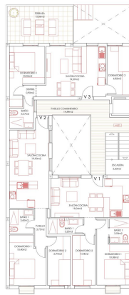
PLANTA PRIMERA
